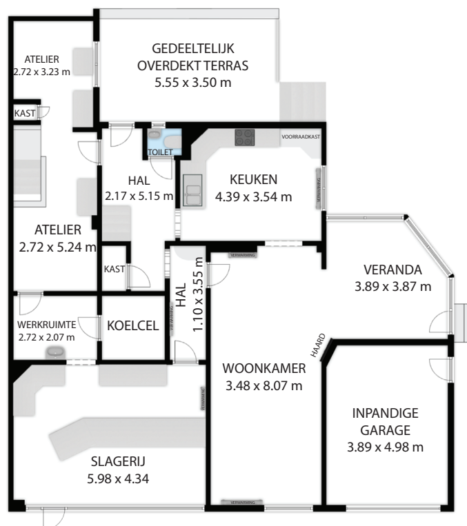
GELIJKVLOERS
